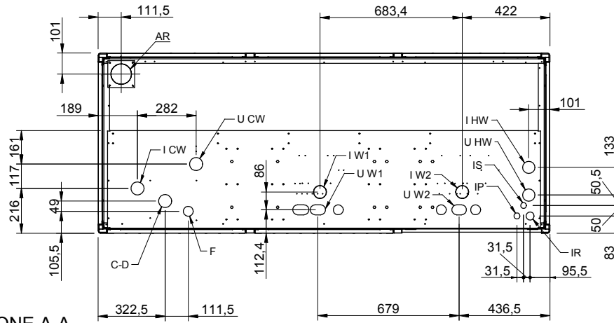
SEZIONE A-A
